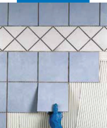
Укладка плитки ординарного обжига на штукатуренную стену в ванной
